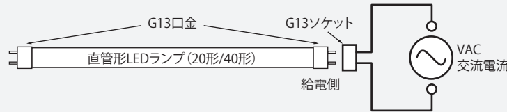
【ELNシリーズ 結線図】
